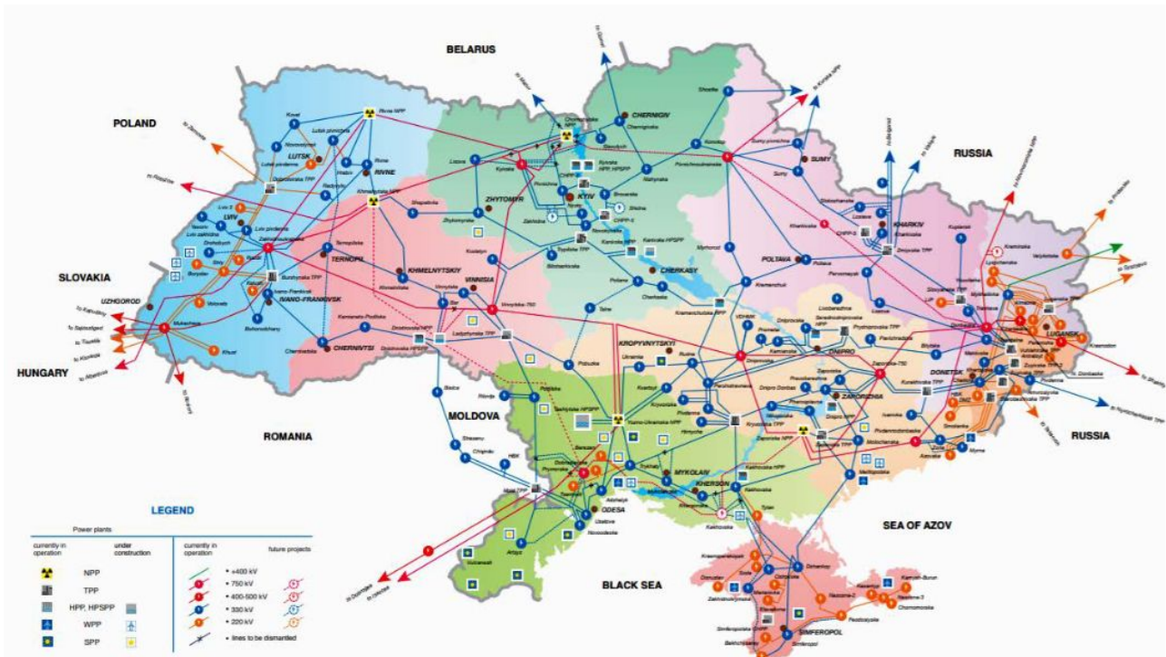
Carte du réseau à haute tension ukrainien en 2019 avec sources de production ( NPP : nucléaire - TPP : thermique - HPP/HPSP : cogénération - WPP : éolien - SPP : solaire)
